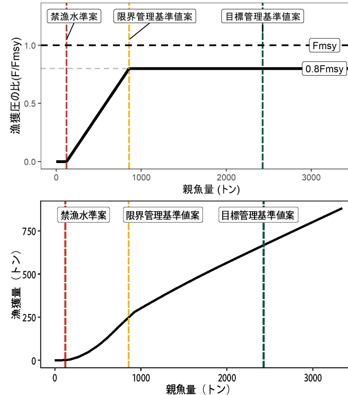
図7 漁獲管理規則案 (上図：縦軸は漁獲圧、下図：縦軸は漁獲量)
