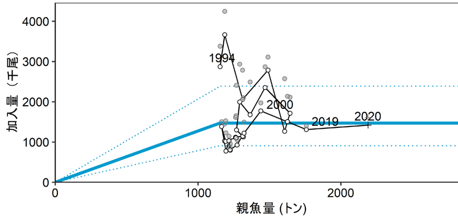
図4 再生産関係
