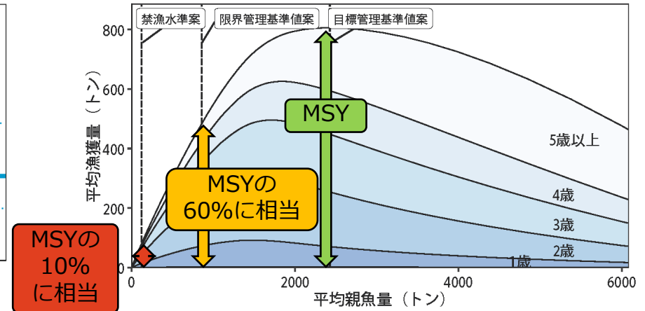
図5 管理基準値案と禁漁水準案
