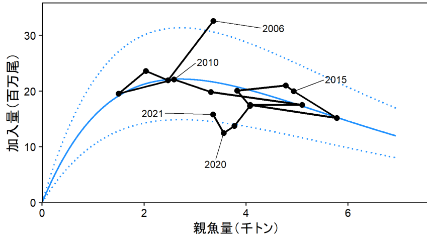
図4 再生産関係
