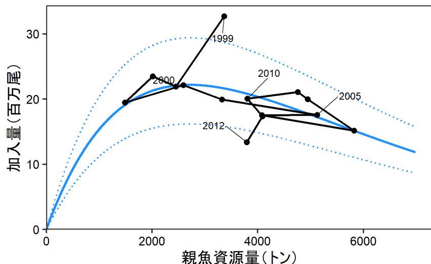
図4 再生産関係
