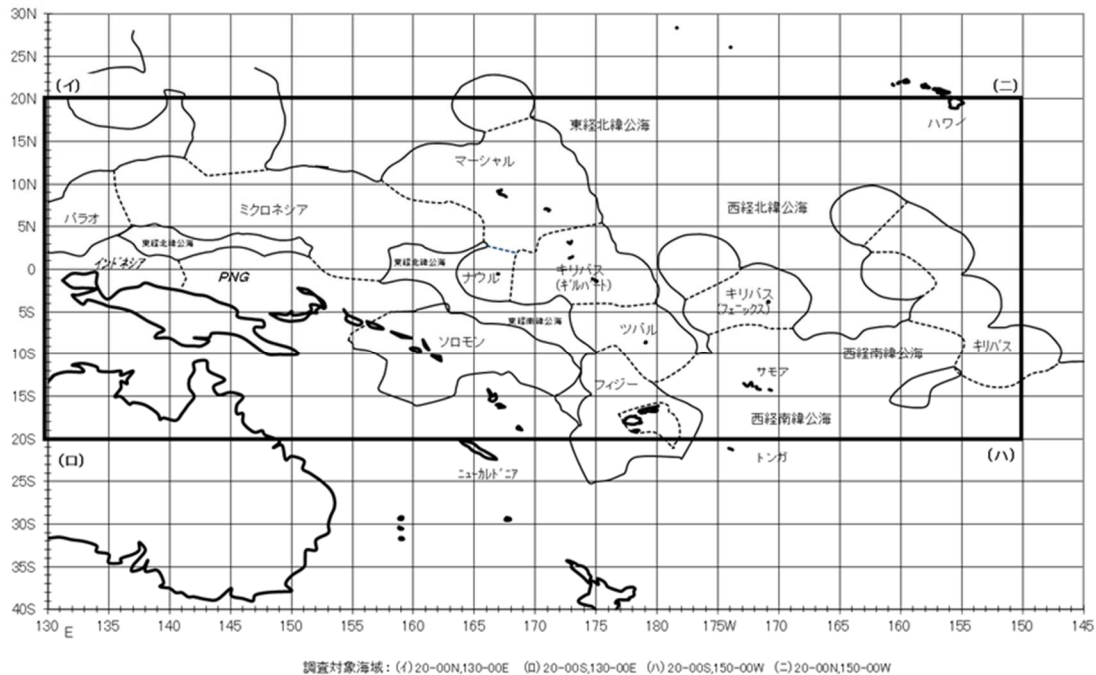
図1 調査対象海域（熱帯太平洋海域）
